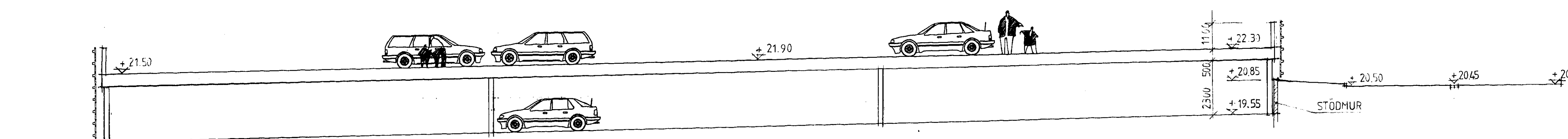
SEKTION A-A 1:100
